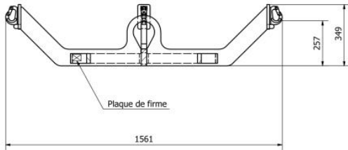
B-B ( 1 : 10 )
